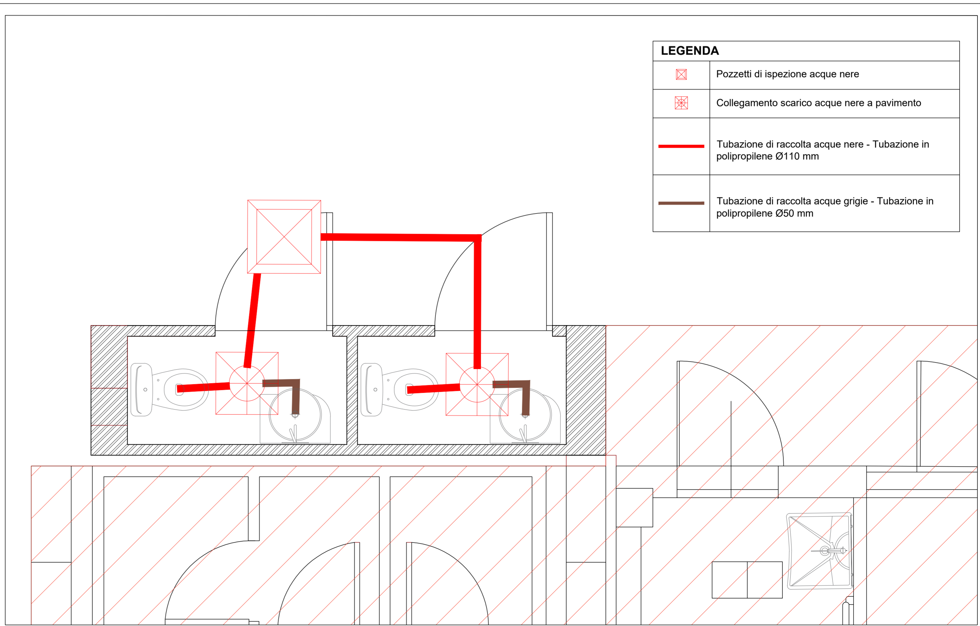
Impianto idrico sanitario
